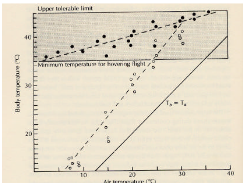
Figuur 8. Lichaamstemperatuur ( T_b ) van thorax (gesloten rondjes) en abdomen (open rondjes) van een aantal koninginnen ( Bombus vosnesenskii ) die continu vliegen uitgezet tegen de omgevingstemperatuur ( T_a ). Het gearceerde gedeelte geeft de temperatuur van de thorax aan waarbij de hommels kan vliegen (uit: Heinrich, 1979).
