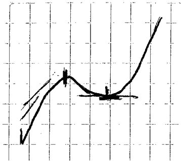
Figuur 6.10.4 Schets van de grafiek van de derdegraads kostenfunctie (I-2)
