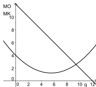
Figuur 6.1.3 Plot van TO' en TK' (I-4)
